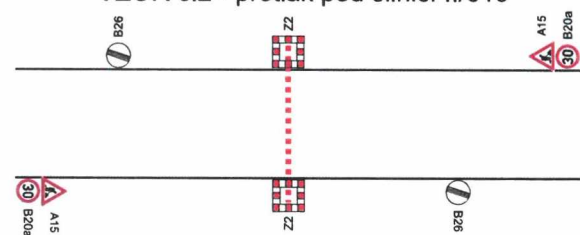
VZOR č.2 - protlak pod silnicí II/610
