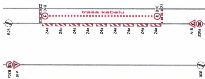
VZOR č.1 - výkop v chodníku
