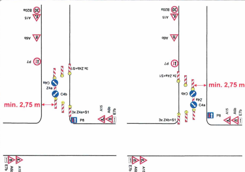
VZOR č.3 - překop po půlkách místní komunikace
