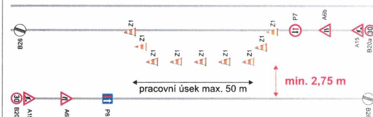
VZOR č.4 - krátkodobý (mobilní) zábor komunikace
